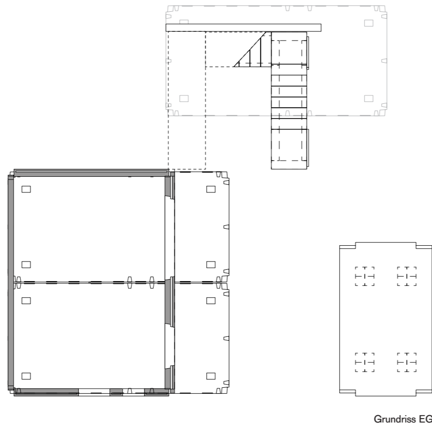
Grundriss EG
